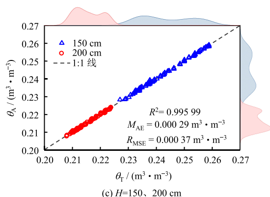
图5 体积含水率模型预测值 \theta_A 和TDR传感器测量值 \theta_T 的比较
