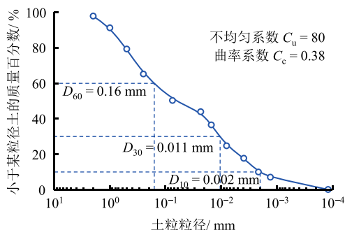
图 2 黄土颗粒级配曲线
