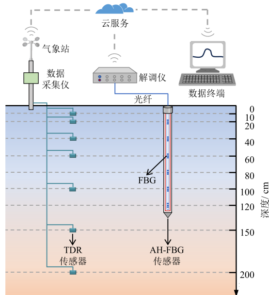
图 3 原位监测系统布设示意图
