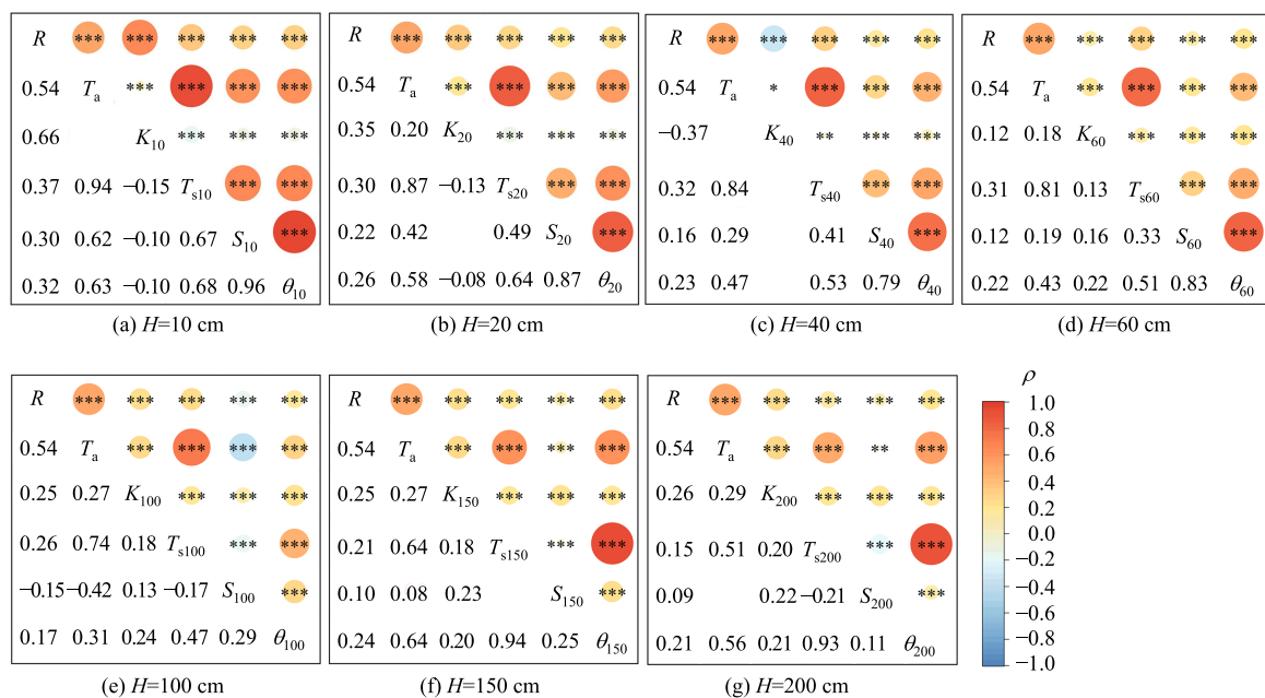
图 4 不同深度处各变量间斯皮尔曼相关系数
