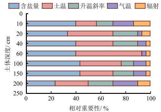
图6 模型输入变量相对重要性 Fig.6 Relative importance of model variables
