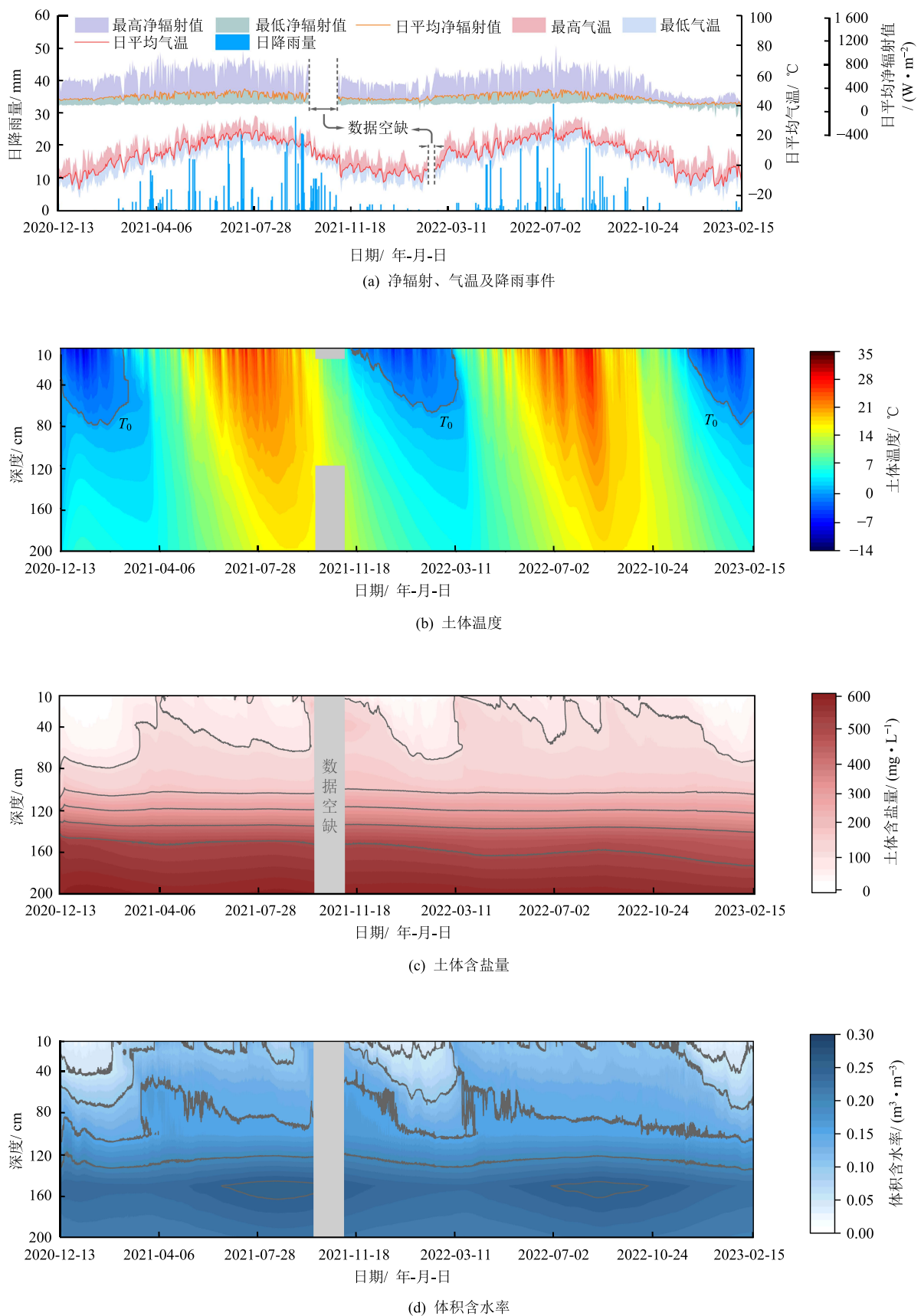
图8 气象记录及地下多物理场时空演化
